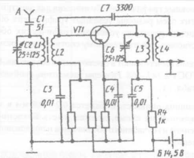
Усилитель высокочастотный
