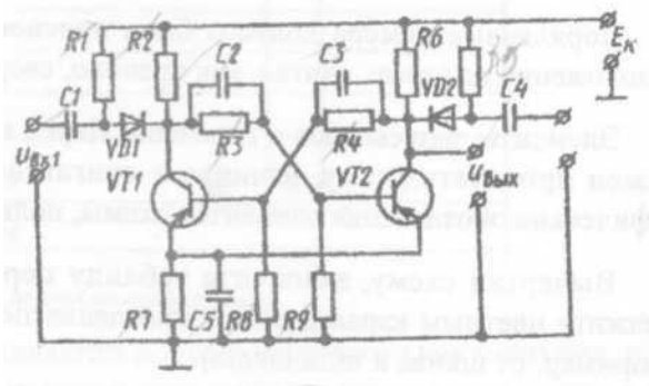
Триггер
