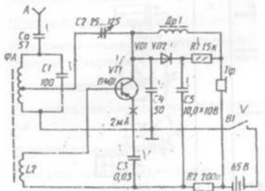
Регенераторный приемник
