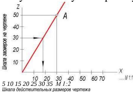
Рисунок 1 - Построение углового масштаба
