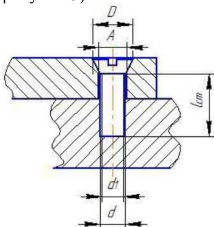
Рисунок 3 - Упрощенное соединение винтом ГОСТ 17475-80
