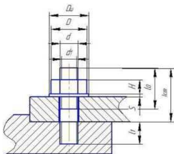
Рисунок 2 - Упрощенное соединение шпилькой 8. Произвести расчет соединения винтом, в соответствии с заданием, по формулам:
