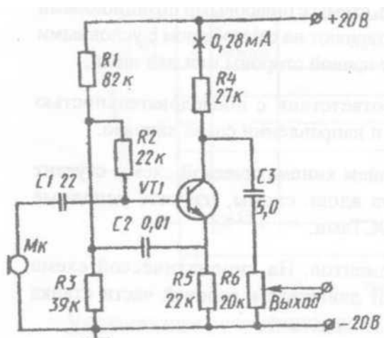
Предварительный усилитель
