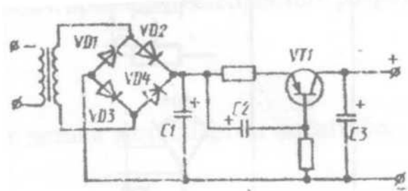
Стабилизатор напряжения
