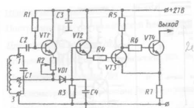
Усилитель высокочастотный
